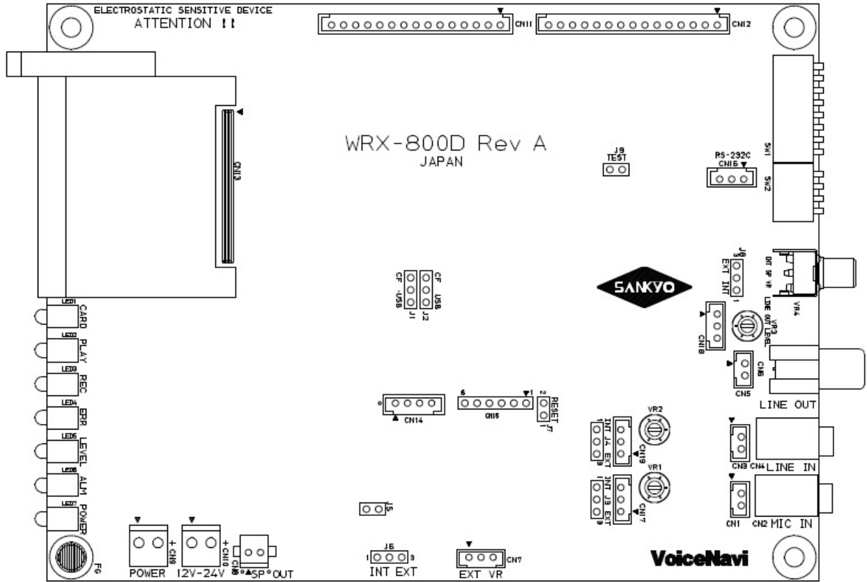
【上面図】
