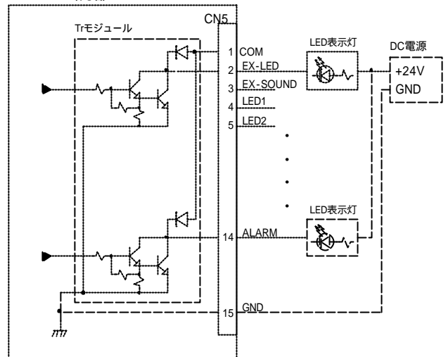
FVA820 出力部
