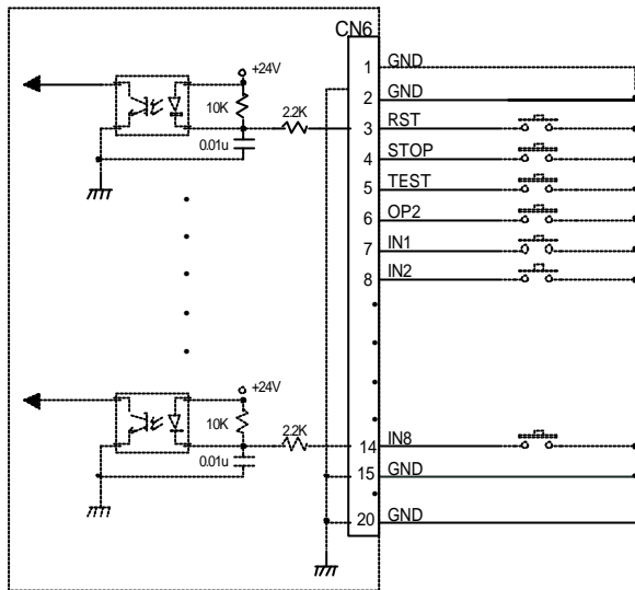
FVA820 入力部
