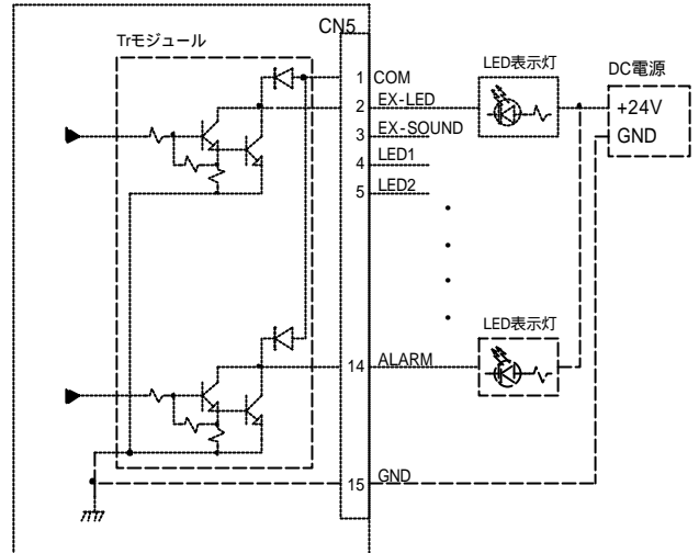
FVA820 出力部
