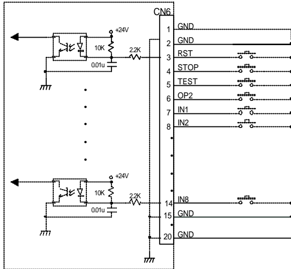
FVA820 入力部
